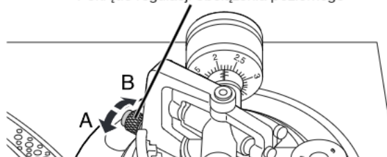
Pokrętło regulacji obciążenia poziomego
